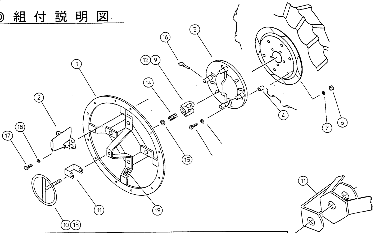
⑪取付詳細
