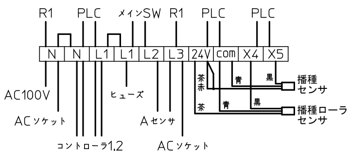
端子台配線図
