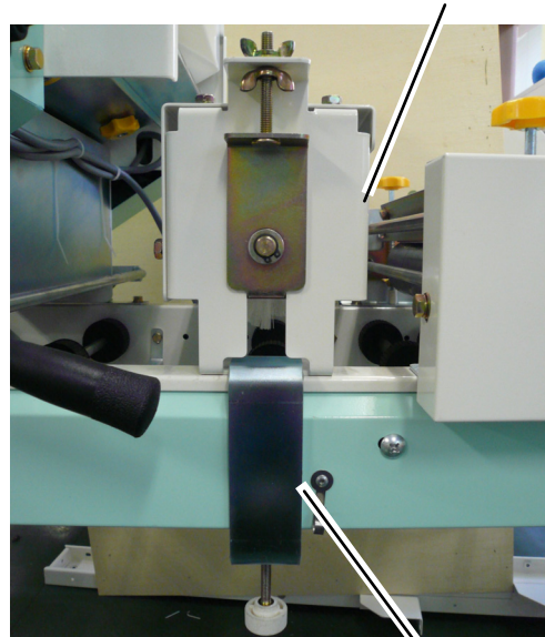
籾落とし回転ブラシ BC9
