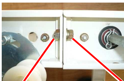
六角ナット(M8)
