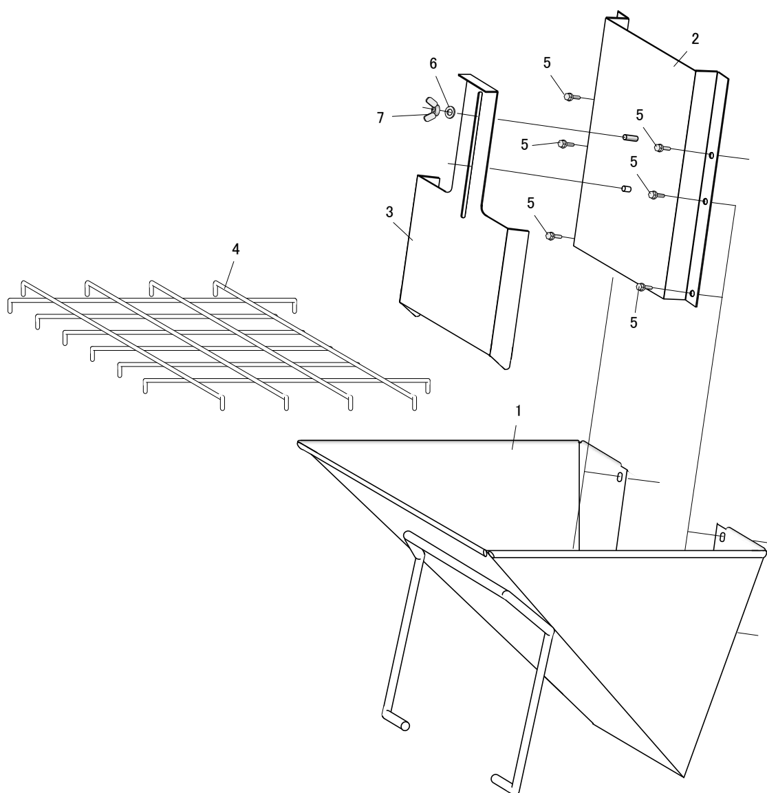
[ ホツパーAssy パーツリスト ]
