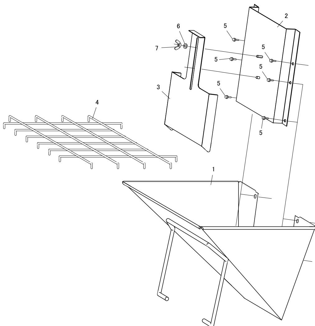
[SCS28・28N ホッパ―Assy パーツリスト]
