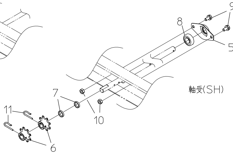
軸受(SG)
