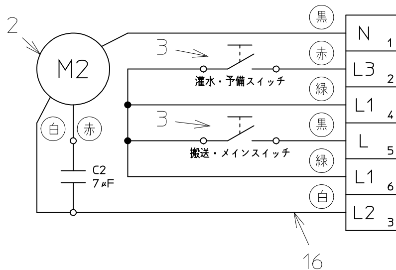
攪拌駆動部結線図
