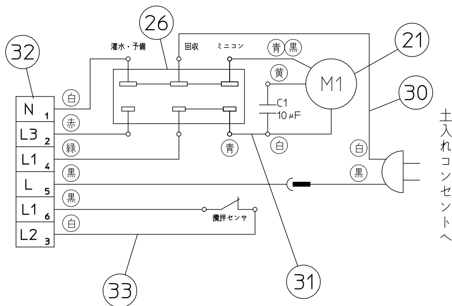
充填駆動部結線図
