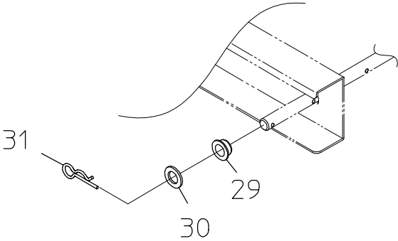
軸受(A)
